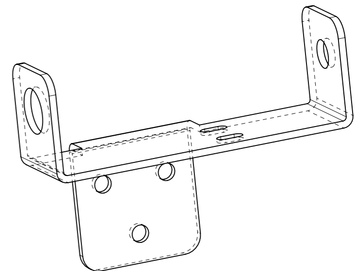
Isometrische Ansicht
